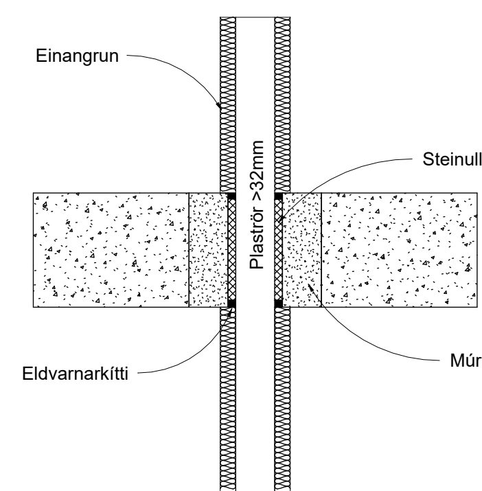
Brunapétting á plastlögn stærri en Ø32mm í gegnum steipt gólf innan lagnaskakts
