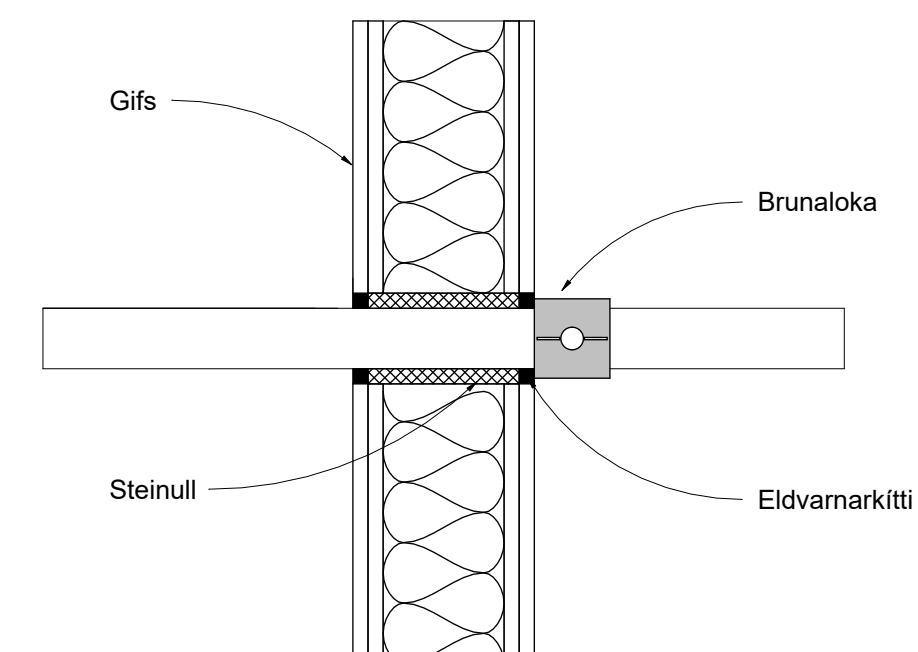
Brunapétting á loftræstilögn í gegnum léttan vegg
